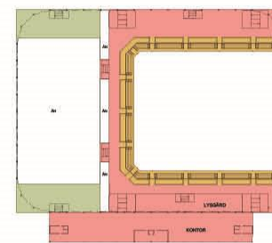
4.etg
